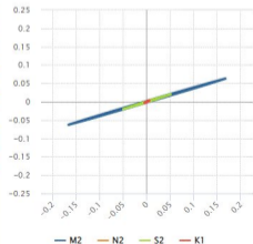
Tidevannsellipser
